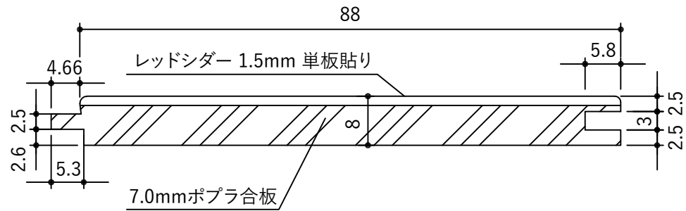
断面図
